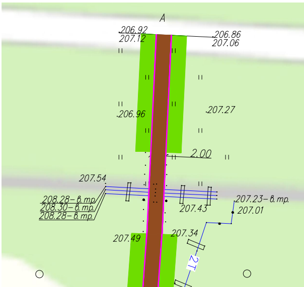
2.Переход через теплотрассу
