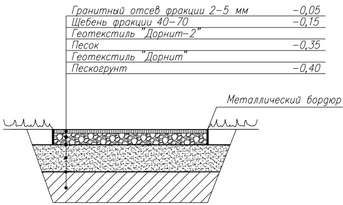
Покрывтие пешеходных дорожек из гранитного отсева Тип-1
