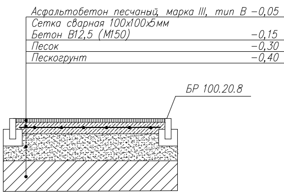
Устройство тротуара из асфальтобетона
